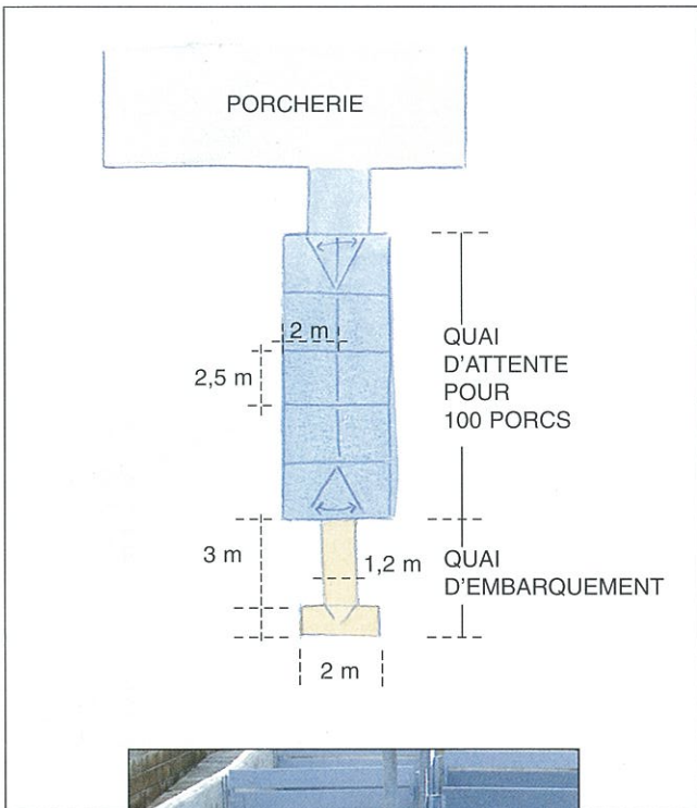
exemple de LOCAL SÉPARÉ DE LA PORCHERIE cases de dimensions fixes
