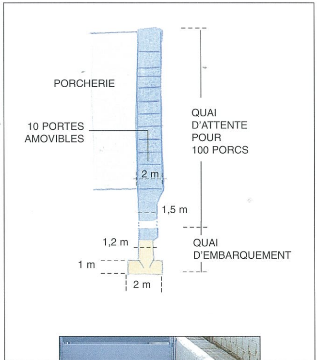
exemple de LOCAL SITUÉ EN CÔTÉ DE LA PORCHERIE cases de dimensions variables. Portes amovibles
