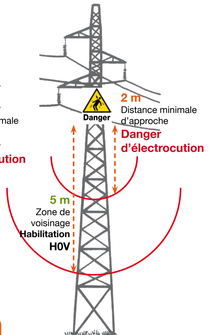
Ligne Haute Tension B (HTB) supérieure à 50 000 V (souvent de 225 à 400 kV)
